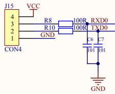
UART接口
