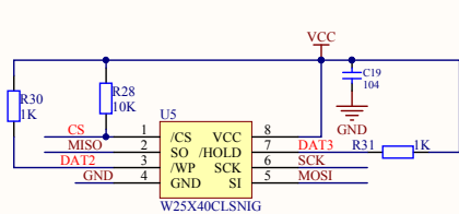
SPI接口电路
