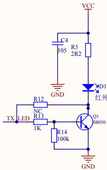
红外发射电路:PC5最大电流500mA
