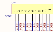
LCD驱动电路:带RTC/电量显示
