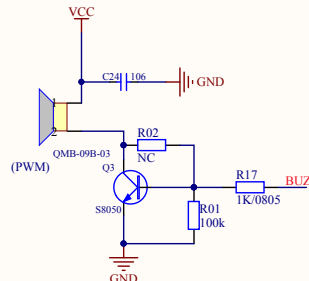
蜂鸣器驱动电路
