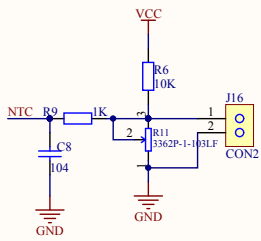
ADC电路
